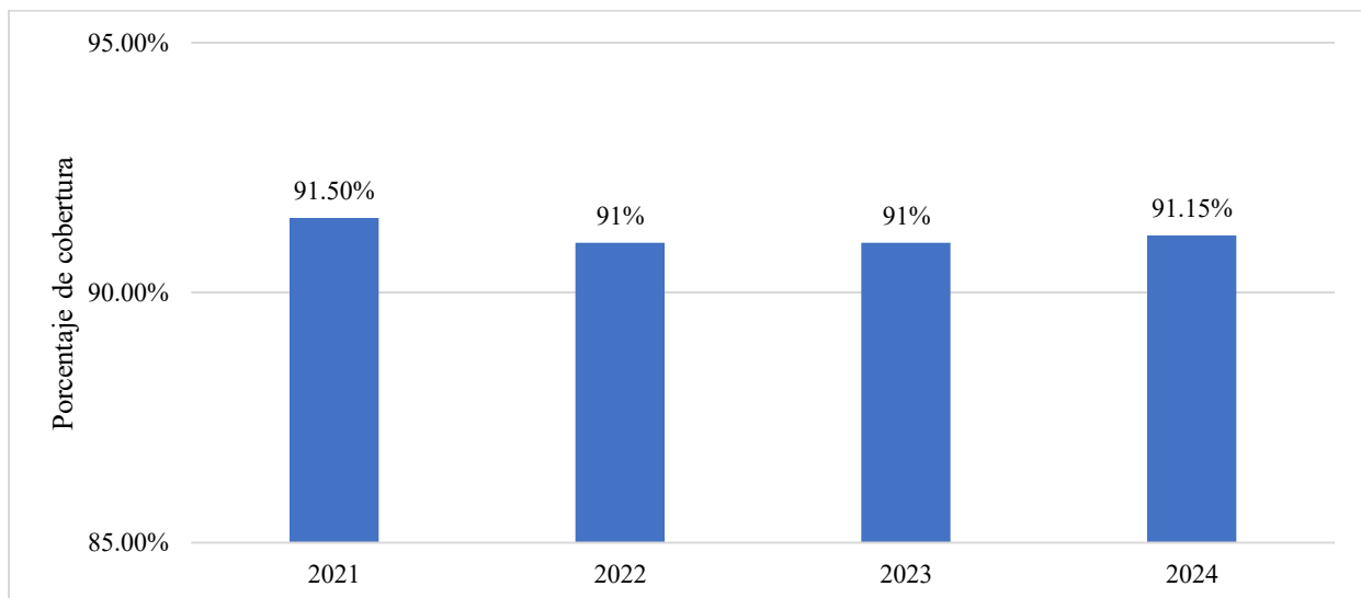
Gráfico 24. Cobertura de alcantarillado en el área de servicio de Aguas de Cartagena
